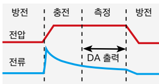
시퀀스 제어
