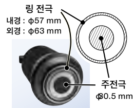
본체 전극 (SM9001 본체 밑면)
