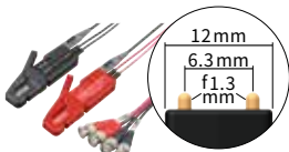
클립형 프로브 L2002 케이블 길이 1.5 m
