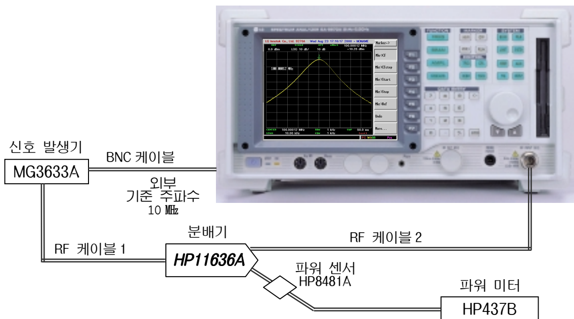
그림 6-8. 주파수 응답
