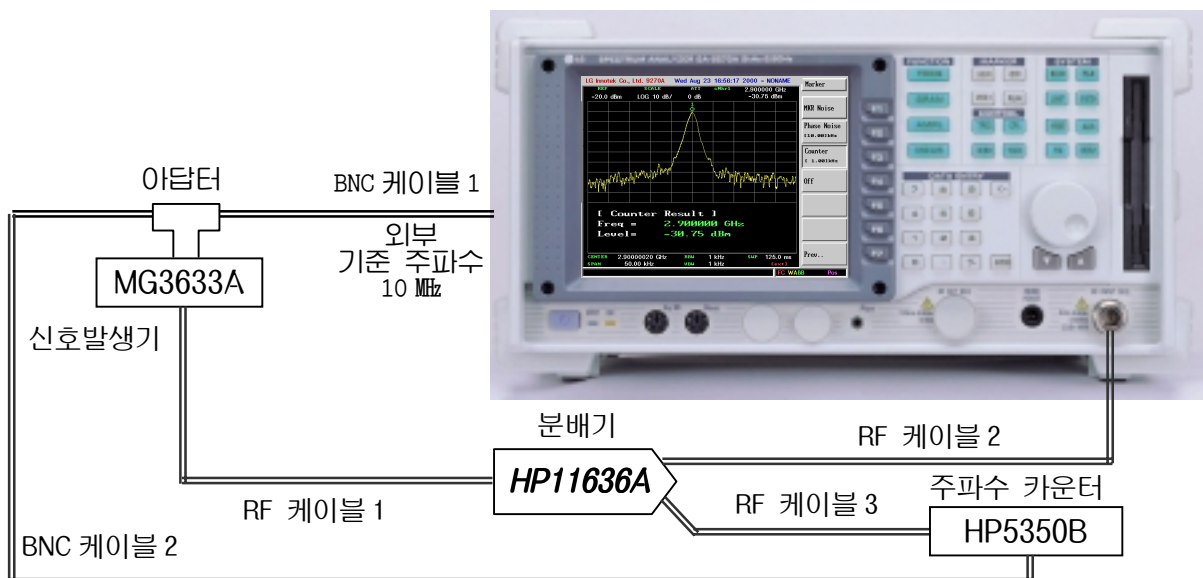
그림 6-6. 마커 카운터 정확도
