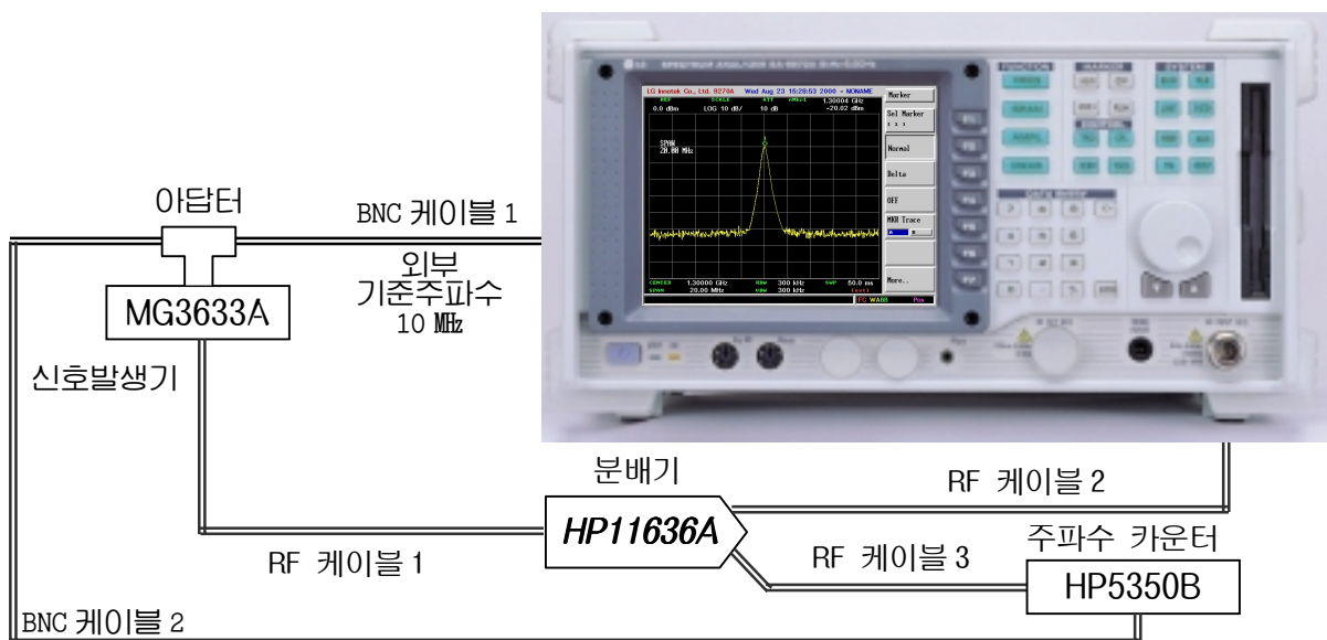
그림 6-2. 주파수 판독 정확도
