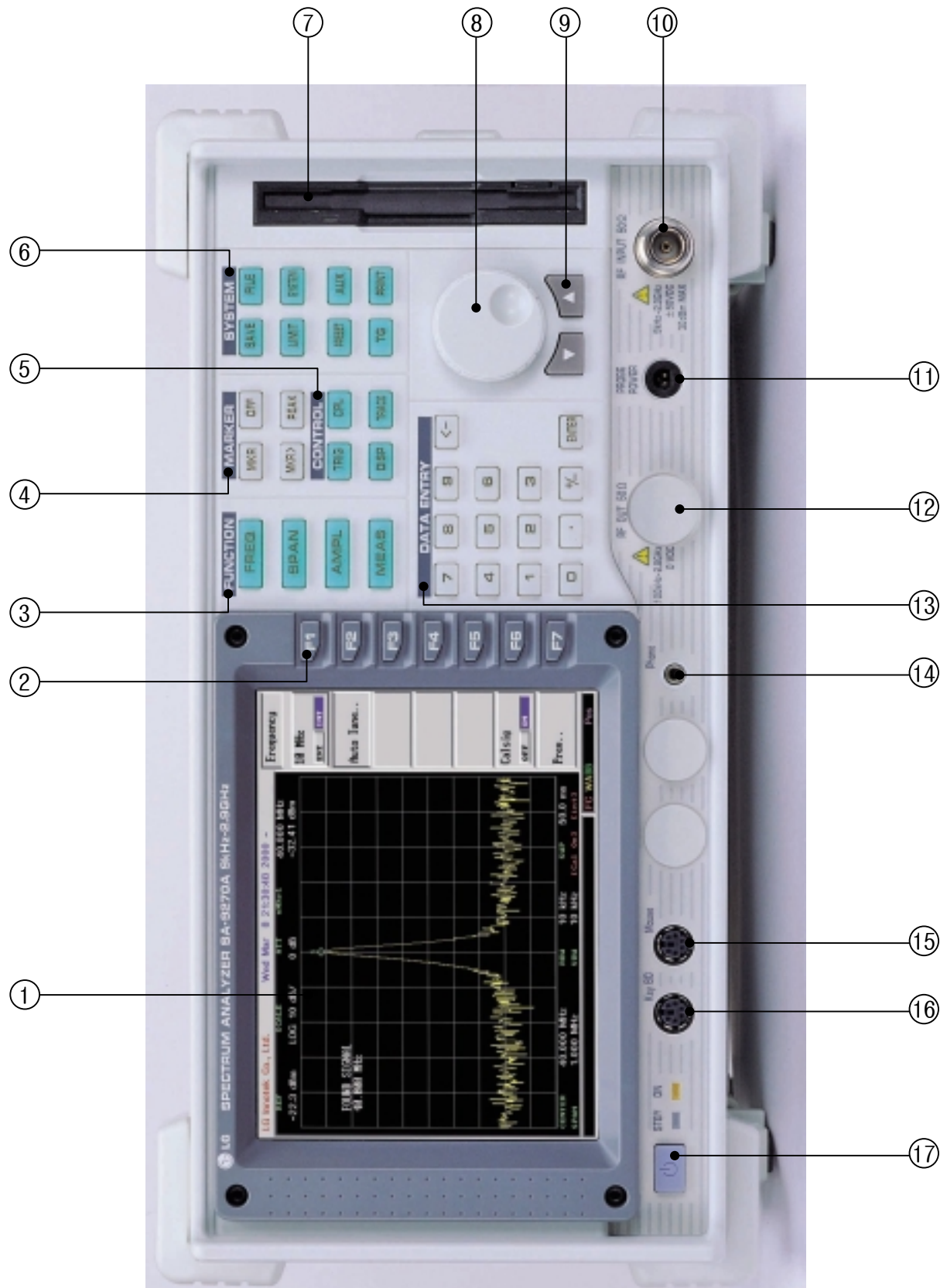
그림 3-1. 전면 패널
