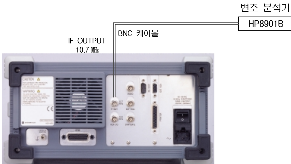
그림 6-13. 잔류 FM 측정도
