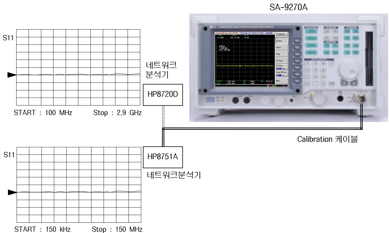
그림 6-17. 입력 VSWR 측정도
