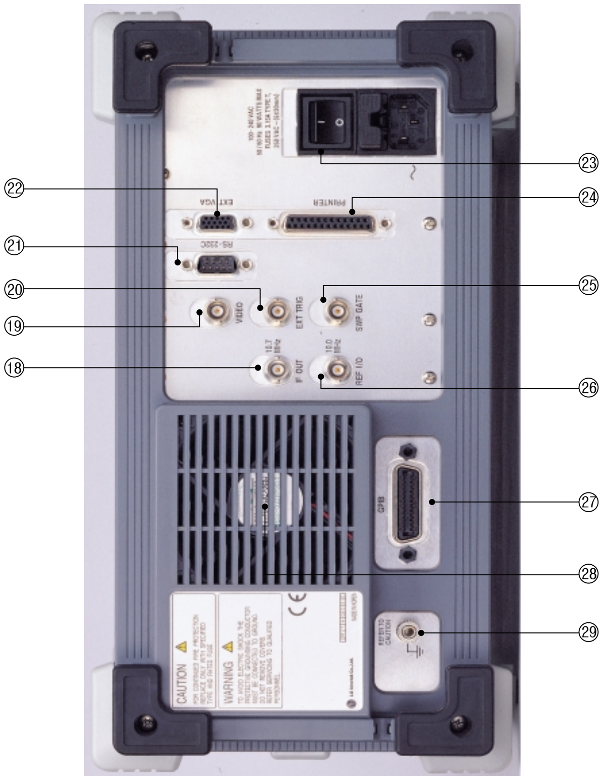
그림 3-2. 후면 패널
