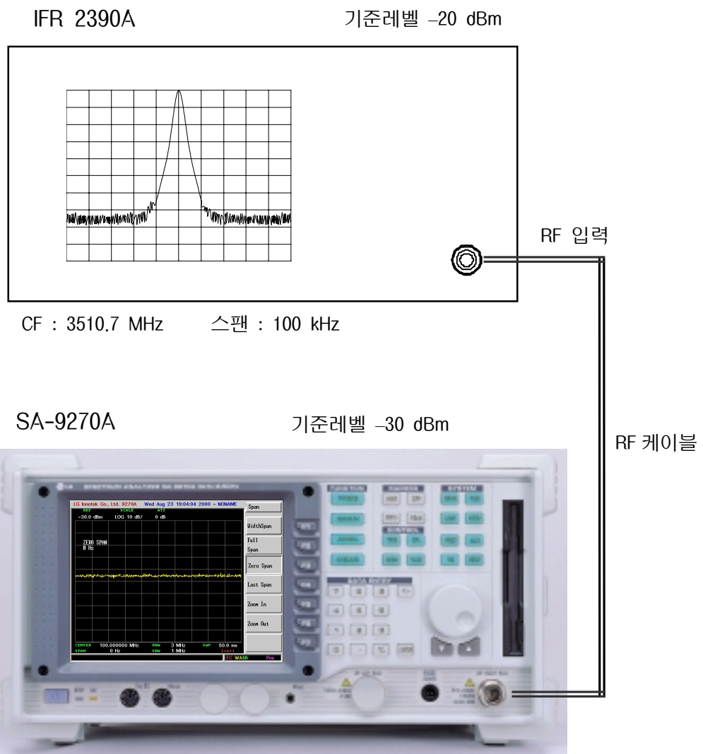
그림 6-16. 국부 방사 측정도
