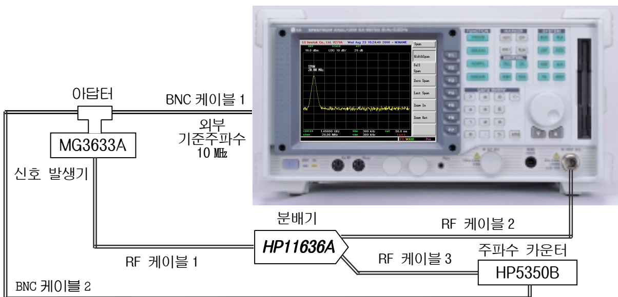
그림 6-3. 주파수 스펙 정확도
