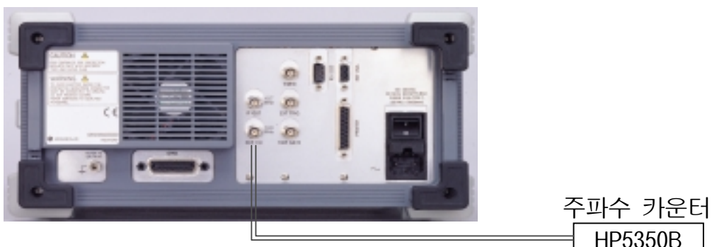
그림 6-1. 기준 발진기 주파수 안정도 시험
