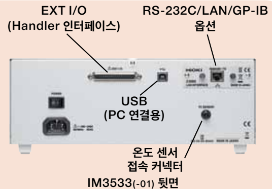
IM3533(-01) 뒷면
