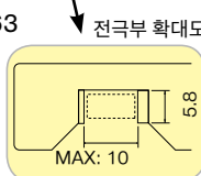
SMD 테스트 픽스처 IM9100
