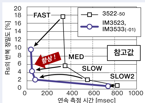
C-D와 ESR 측정 (100kHz)의 연속 측정 시 연속 측정 시간과 Rs의 반복 정밀도 (샘플: 알루미늄 전해 콘덴서 1.5 μF)
