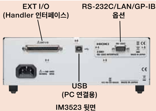
IM3523 뒷면
