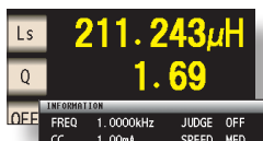
L, Q 표시화면 (1 kHz, CC 1 mA 측정)
