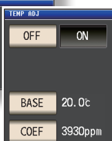
온도 보정 설정 (확대)
