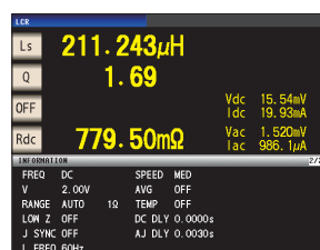
L, Q, Rdc 연속측정화면 L, Q (1 kHz, CC 1 mA 측정)와 Rdc (DC 측정)의 표시화면
