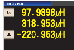
트랜스 측정 모드 인덕턴스 차 측정 화면
