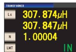
트랜스 측정 모드 권수비 측정 · 판정 화면
