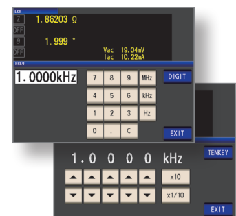
주파수 설정 (10개 버튼 입력과 업 다운 입력)
