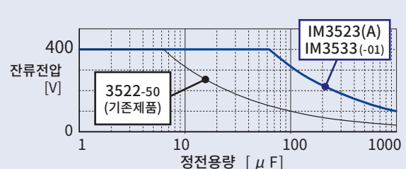
LCR 미터를 보호할 수 있는 정전용량과 잔류전압의 관계
