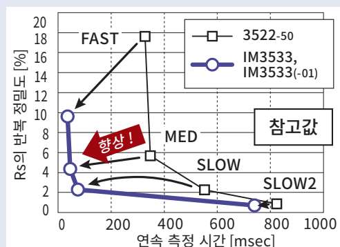
C-D와 ESR 측정 (100kHz)의 연속 측정 시 연속 측정 시간과 Rs의 반복 정밀도 (샘플: 알루미늄 전해 콘덴서 1.5 μF)
